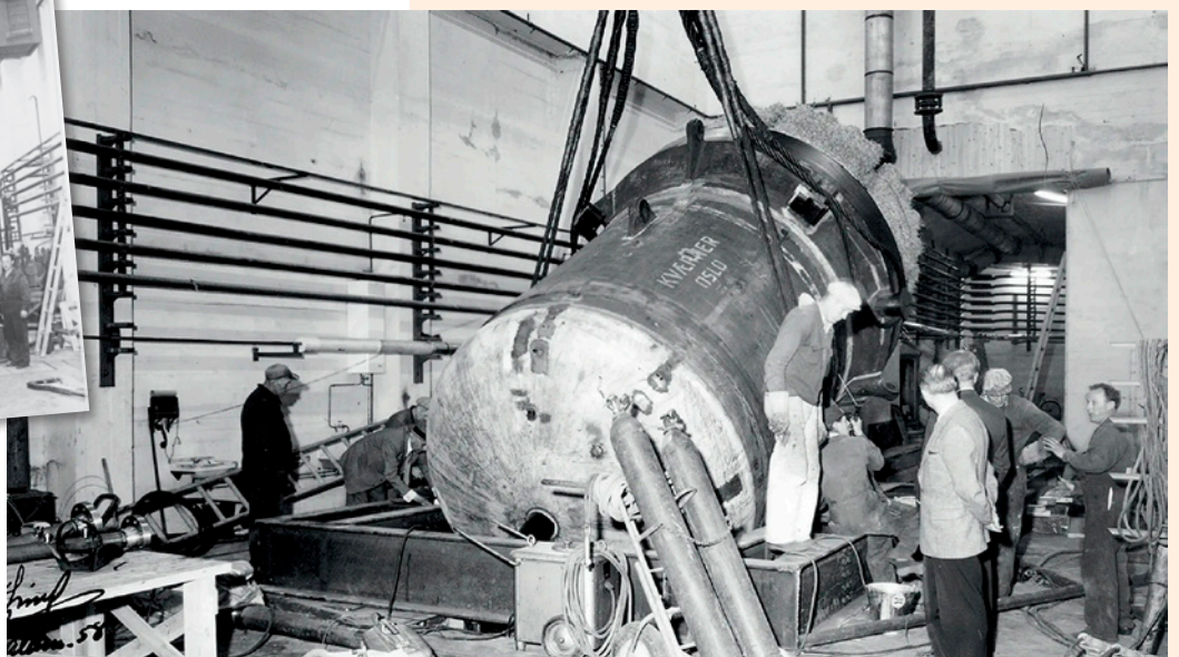
Reaktortanken som heises på plass i Halden. På reaktortanken kan vi se «Kværner» inngravert. Foto: IFE
