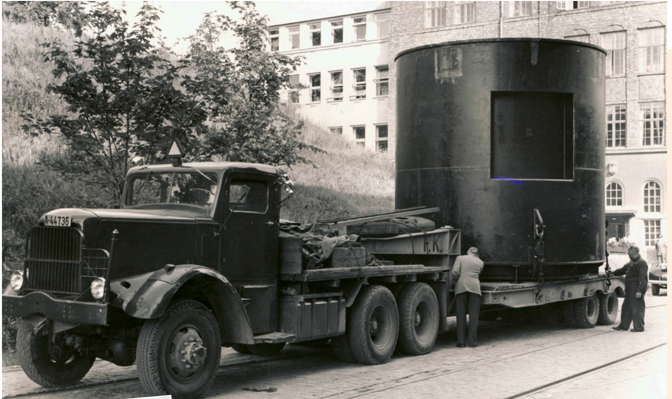
Når man skulle bygge reaktor i Norge var det fokus på synergier i industrien. Reaktortanken til Haldenreaktoren ble bygget av Kværner Brug AS. Foto: IFE
